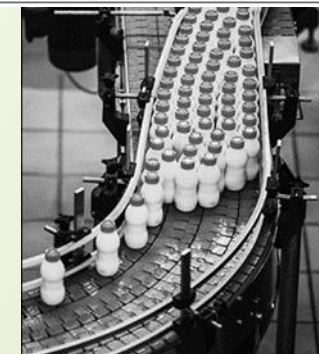
Лінія з виробництва молочного дитячого харчування торгової марки «Агуша» компанії «Вімм-Білл-Данн Україна»
